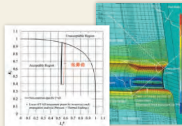
FEM解析と 自社材料データによる 圧力容器の余寿命評価
